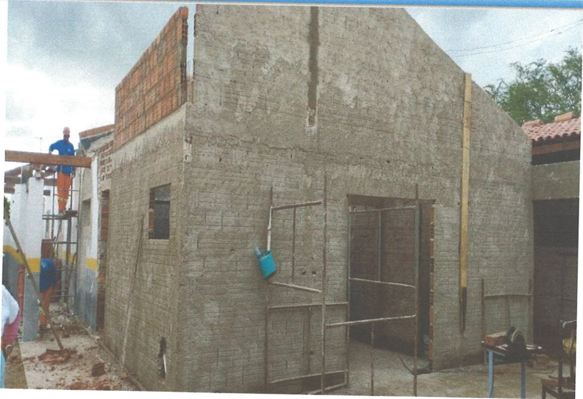
FOTO 09 EXECUÇÃO DE CHAPISCO E INSTALAÇÃO DE TESOURAS DE MADEIRA NA COBERTURA
