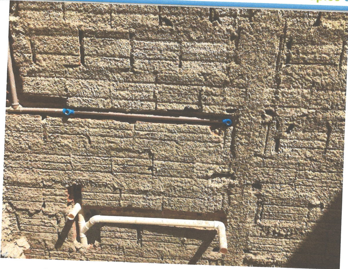
FOTO 14 EXECUÇÃO DE PONTOS DE AGUA E ESGOTO NOS BANHEIROS
