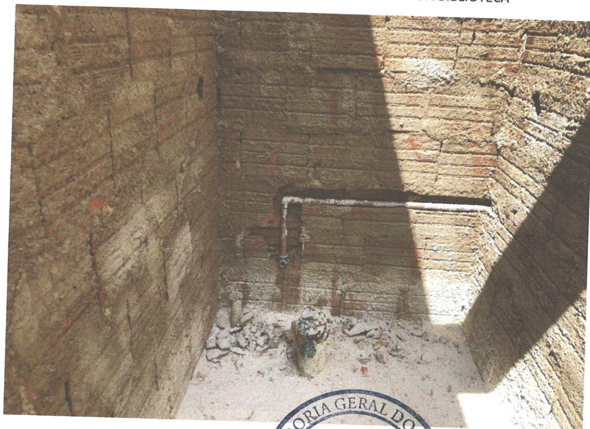
FOTO 12 EXECUÇÃO DE PONTOS DE AGUA NOS BANHEIROS
